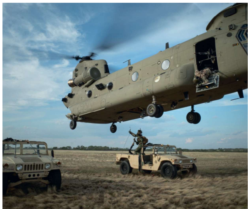
Aanhaken van een US HUMVEE aan een CH-47
